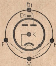
Sockelschaltung
